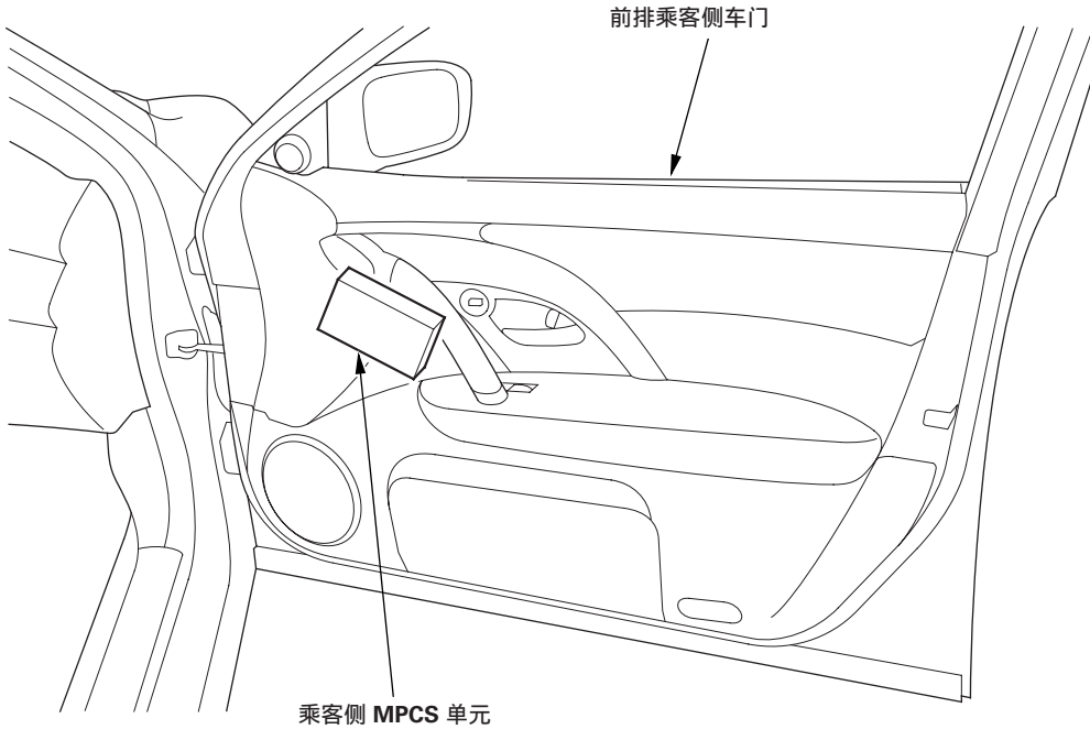
图示为左驾车型，右驾车型与此相似。
